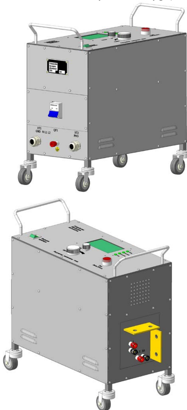
Rys. Nr 1. Wygląd zewnętrzny urządzenia
