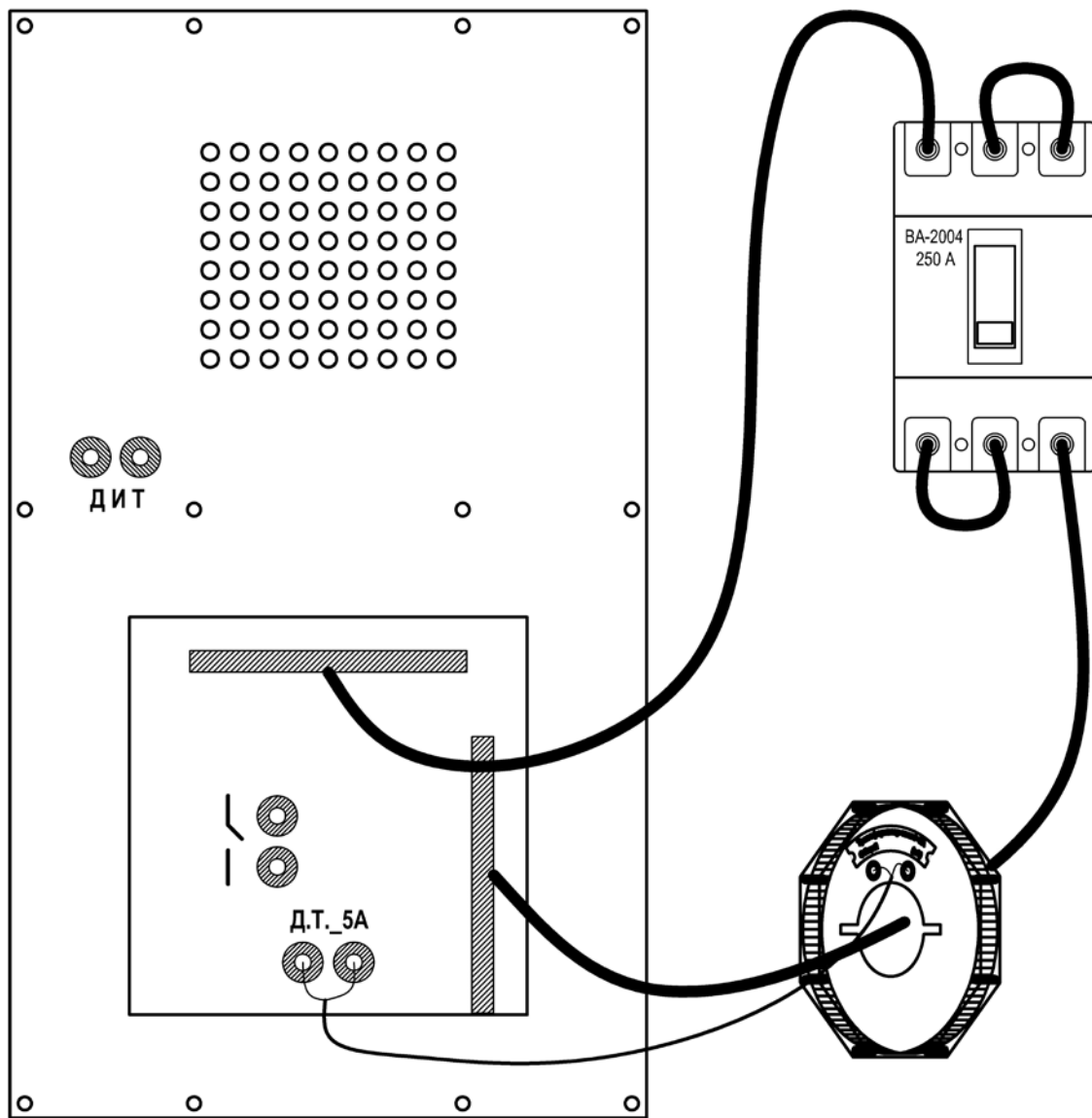
Схема функциональная поверки трехполюсных автоматических выключателей (вариант №2)
